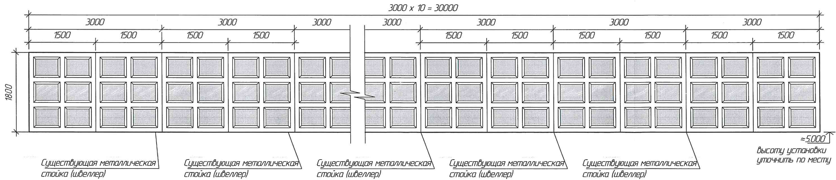
Схема окон главного фасада
