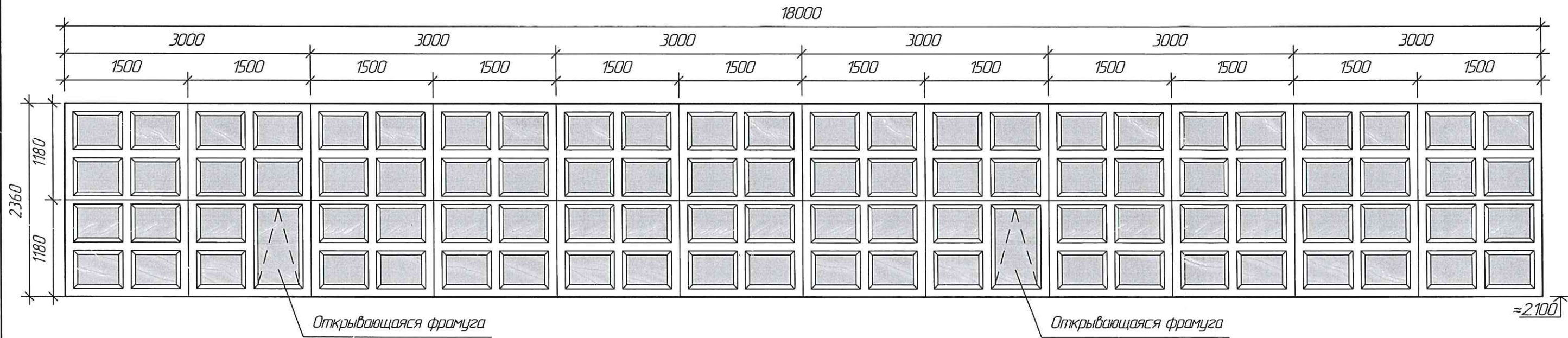
Схема окон бокового фасада (справа)
